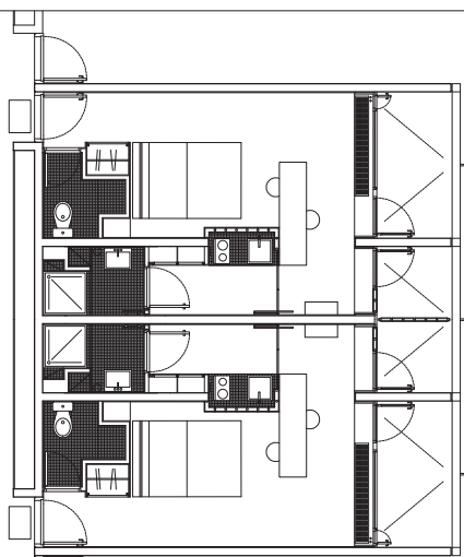
PLAN CHAMBRE TYPE 2
