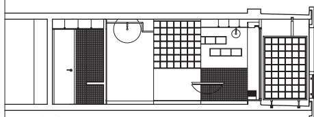
COUPE CHAMBRE TYPE 1
